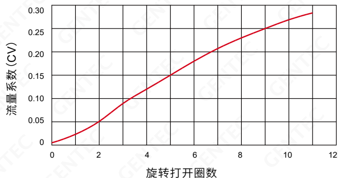
MV30 旋转打开时的流量系数
