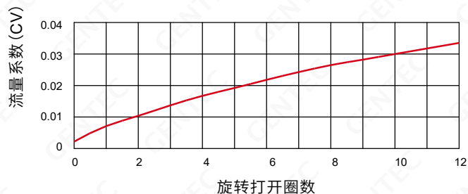
MV31 旋转打开时的流量系数
